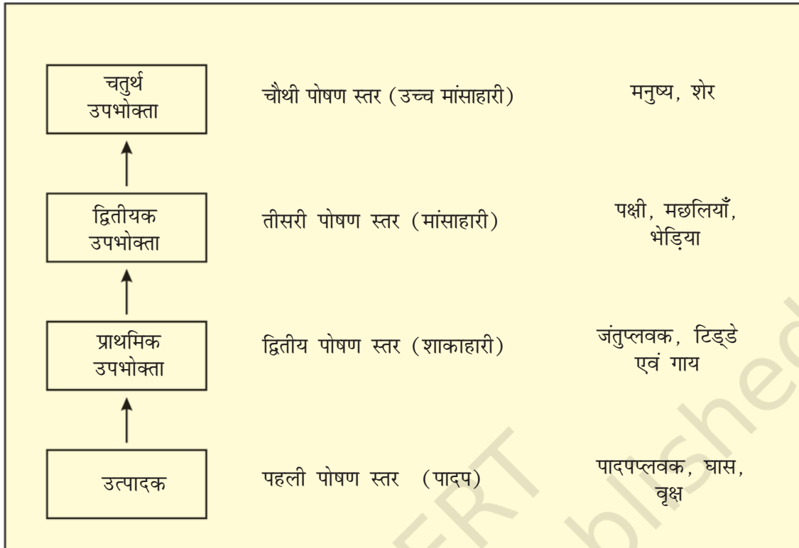
चित्र 12.2 एक पारिस्थितिक तंत्र में पोषण स्तर का आरेखीय निरूपण
